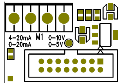
Particolare morsetti di collegamento uscite analogiche
